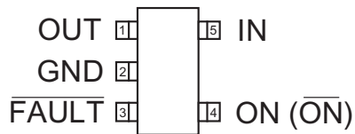
SOT23-5
