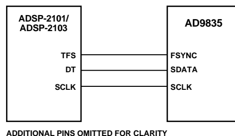
Figure 24. ADSP-2101/ADSP-2103-to-AD9835 Interface
