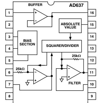
SOIC (R) Package
