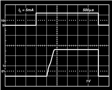
TPC 28. ADR291 Turn-On Time
