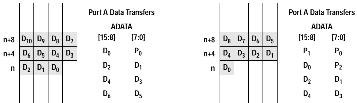
Part (b): One Byte of Padding
