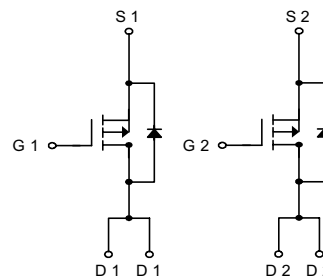
P-Channel MOSFET
