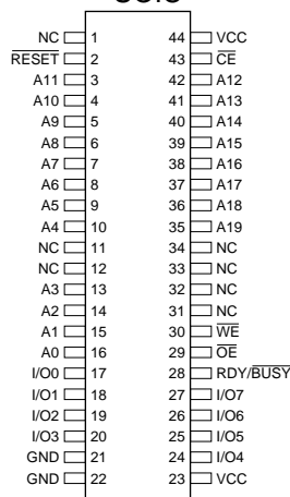
SOIC
