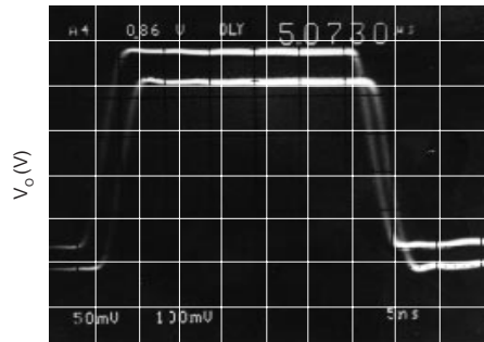
t_R = t_F = 3\text{ns} , V_O = 5\text{Vp-p}
