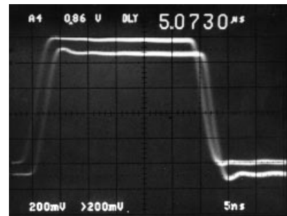
t_R = t_F = 3\text{ns} , V_O = 0.2\text{Vp-p}
