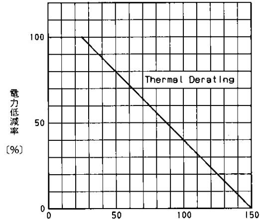
ケース温度 T_c (°C)
