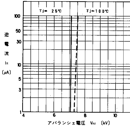
アバランシェ電圧特性 (代表特性) Avalanche Breakdown Voltage
