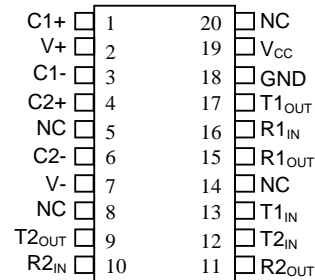
20-Pin TSSOP
