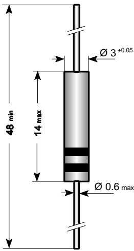
Dimensions / Maße in mm
