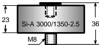
Dimensions / Maße in mm
