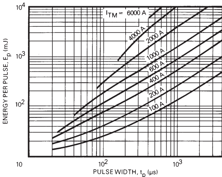
FIG.12 ENERGY PER PER FOR TRAPEZOIDAL PULSES
