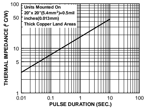
Thermal Impedance
