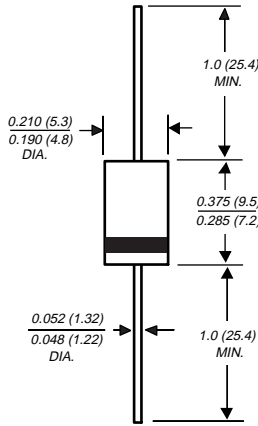
DO-201AD
