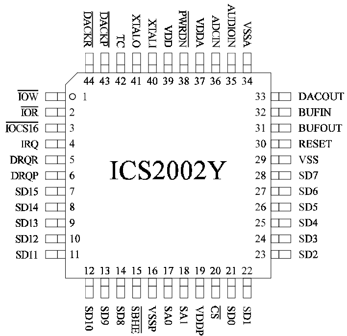
44-Pin TQFP
