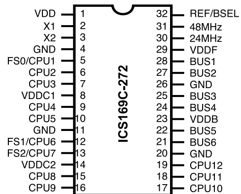
32-Pin SOIC/SOJ
