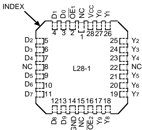
2609 drw 03
