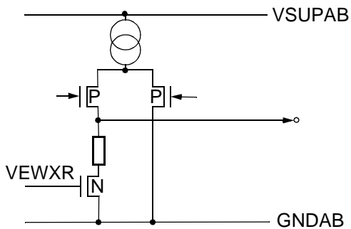
Fig. 3-17: Output pin EW
