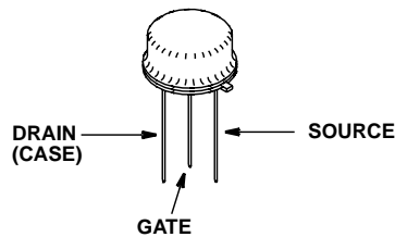
JEDEC TO-205AF
