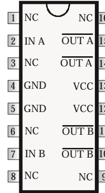
16 Pin SOIC IXDI402SI-16
