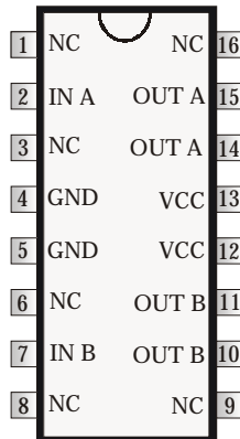
16 Pin SOIC IXDN402SI-16
