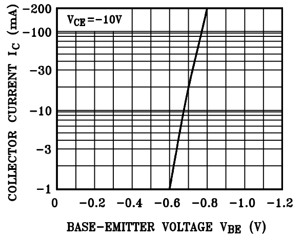
I_C - V_{BE}
