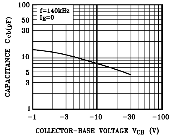
C_{cb} - V_{CB}
