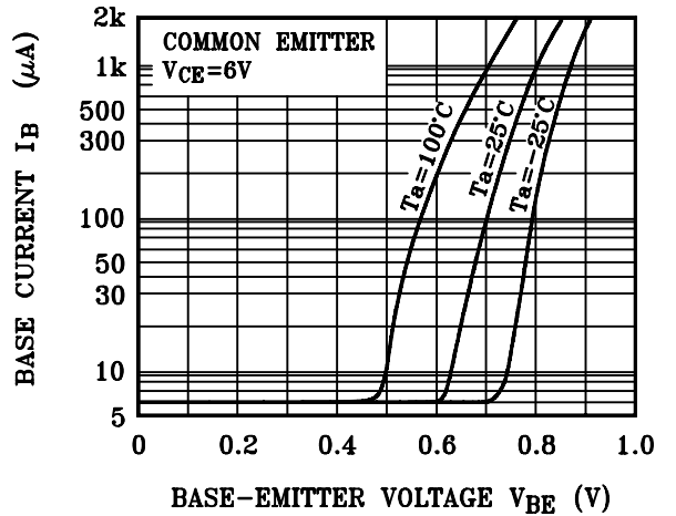
I_B - V_{BE}
