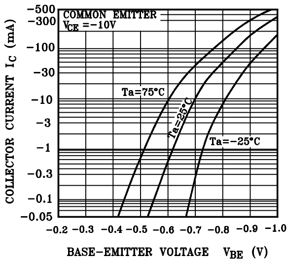
I_C - V_{BE}
