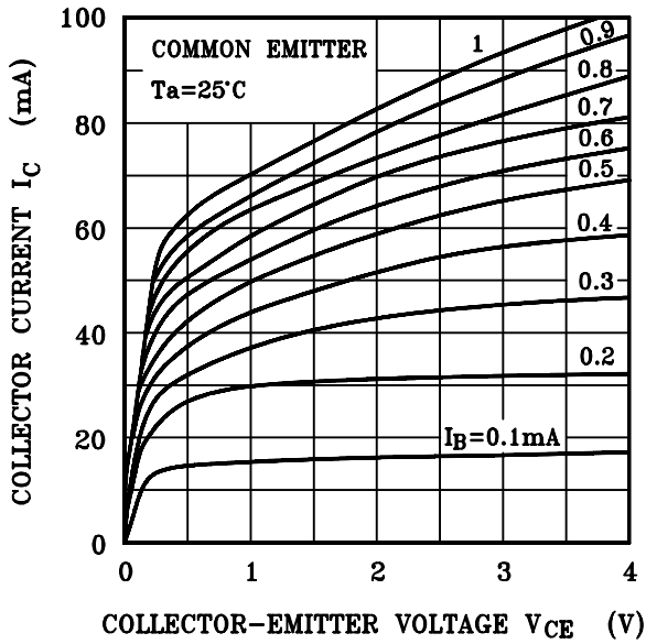
I_C - V_{CE}
