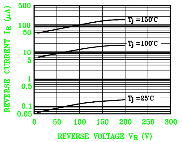
I_R - V_R
