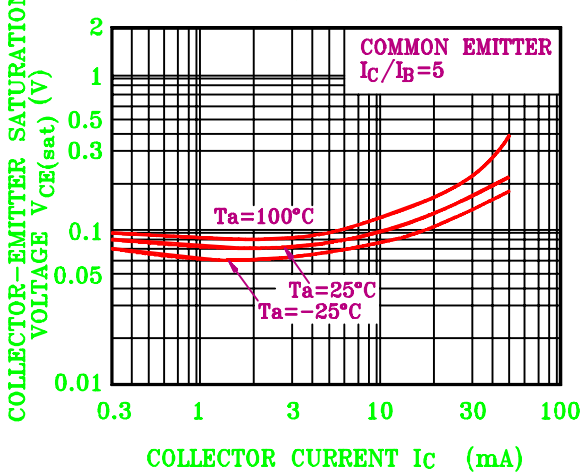
V_{CE(sat)} - I_C
