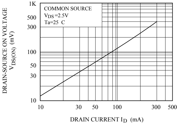
V_{DS(ON)} - I_D
