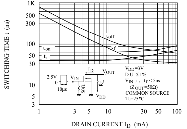
t - I_D
