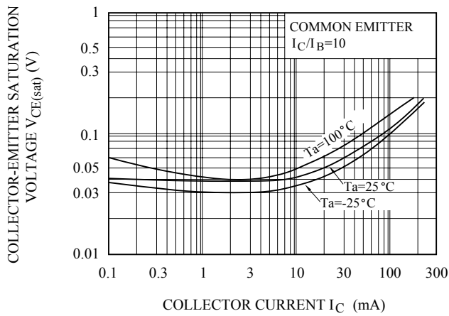
V CE(sat) - I C
