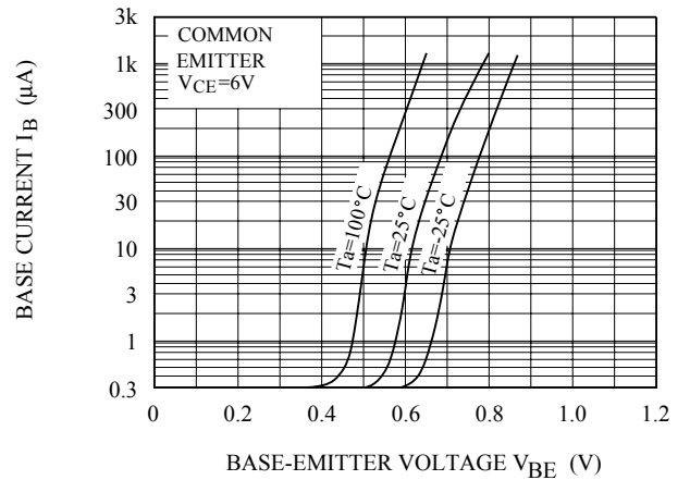
I B - V BE
