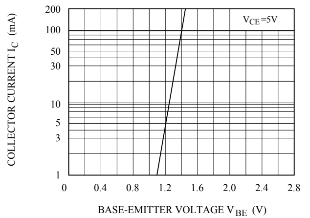
I_C - V_{BE}
