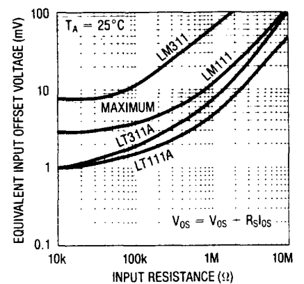
Offset Error
