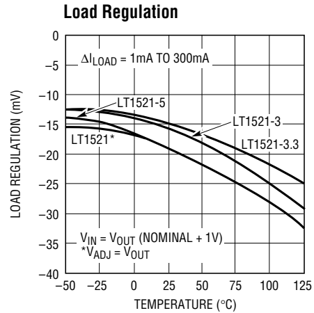
LT1521 • TPC32
