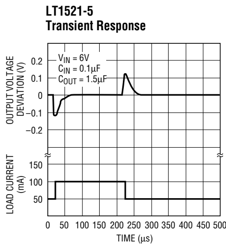
LT1521 • TPC33
