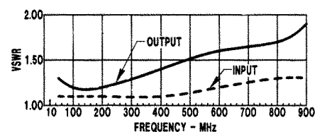
Input/Output VSWR
