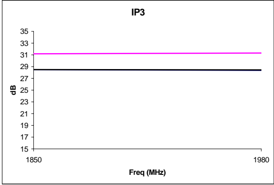
Input IP3
