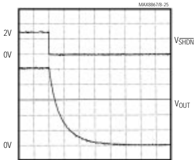
NO LOAD 500 \mu s /div
