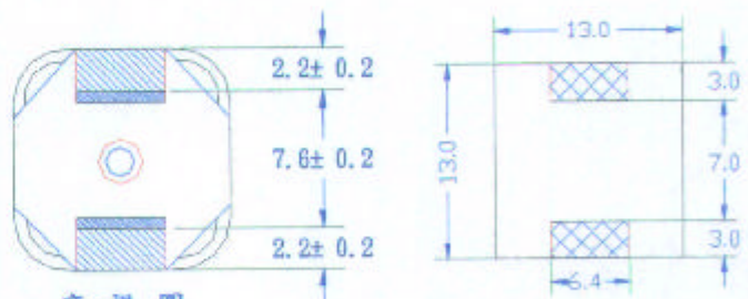
底視圖
