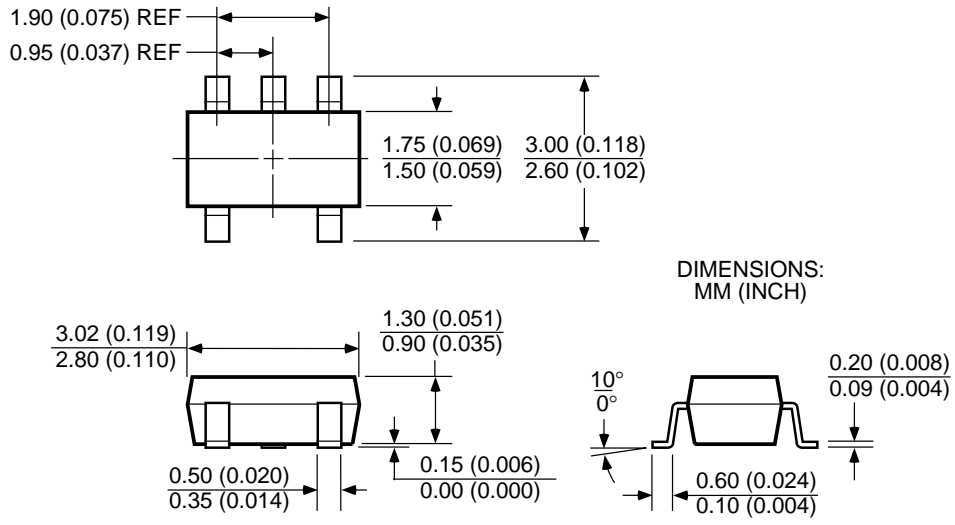
SOT-23-5 (M5)
