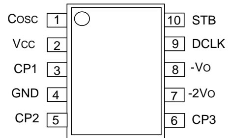
OUTLINE 10P2N
