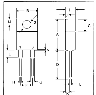
TO-220A
