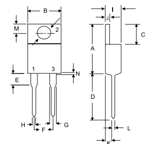
TO-220A
