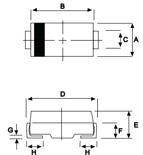
DO-214AC(SMA)
