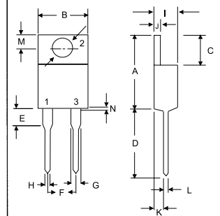
TO-220A
