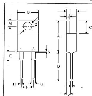
TO-220A
