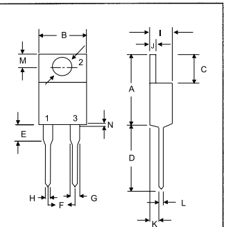
TO-220A
