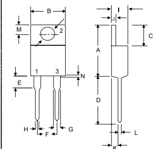
TO-220A
