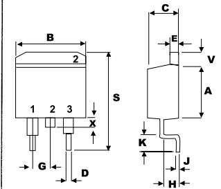
TO-263 (D2-PAK)
