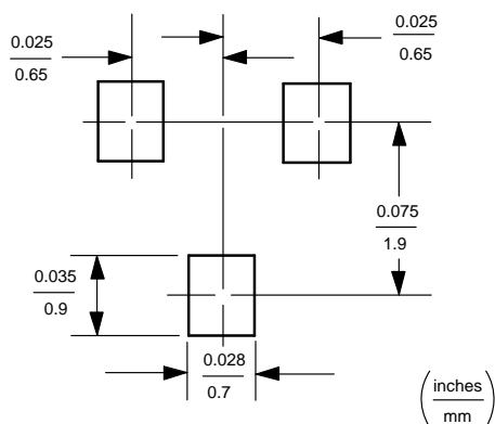
SC-70/SOT-323
