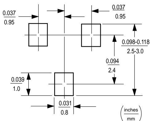
SC-59
