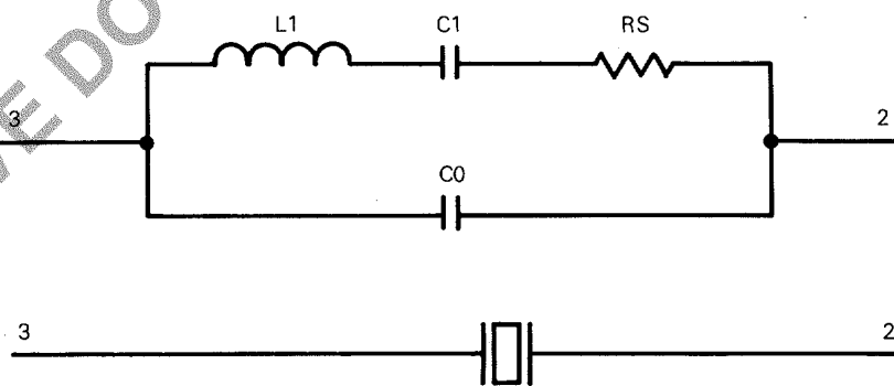
FIGURE 11 — CRYSTAL PARAMETERS
