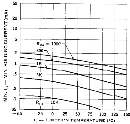
4. Min. Holding Current (Resistor Bias)
